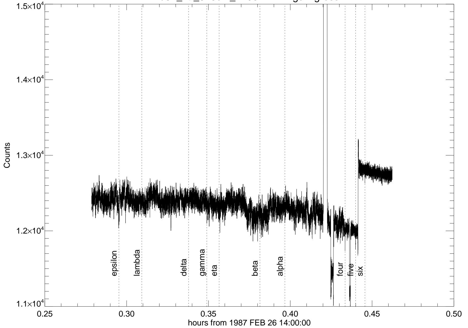
u34_irtf_320cm_2200nm - rings ingress
