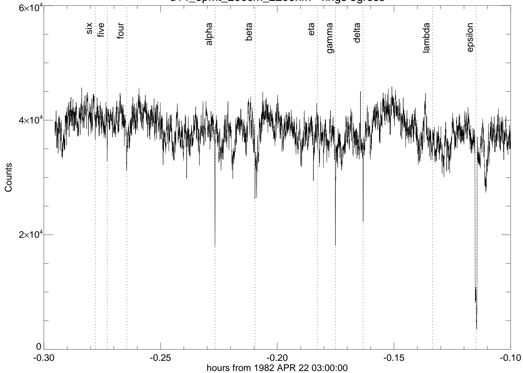
u14_opmt_200cm_2200nm - rings egress
