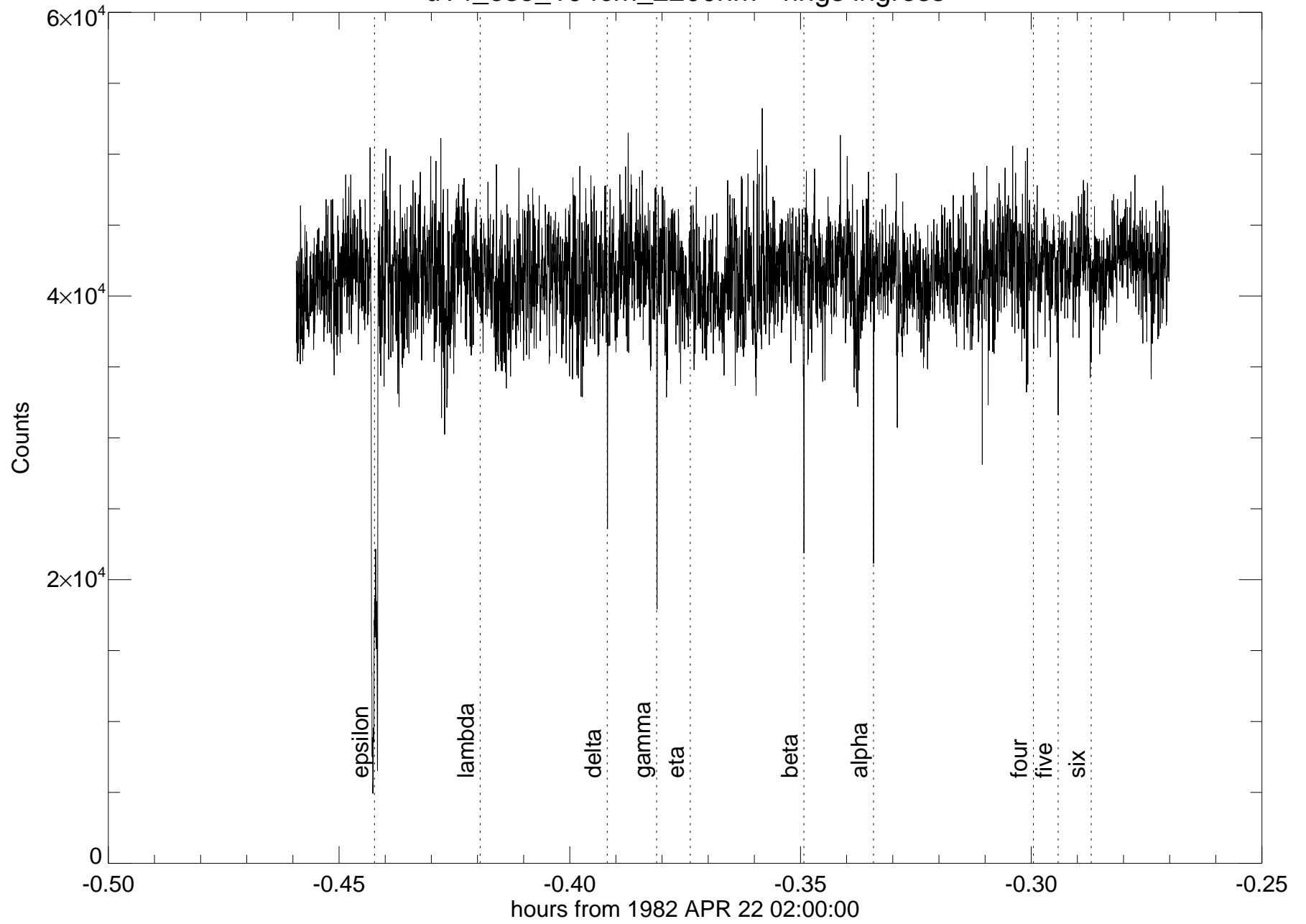
u14_eso_104cm_2200nm - rings ingress
