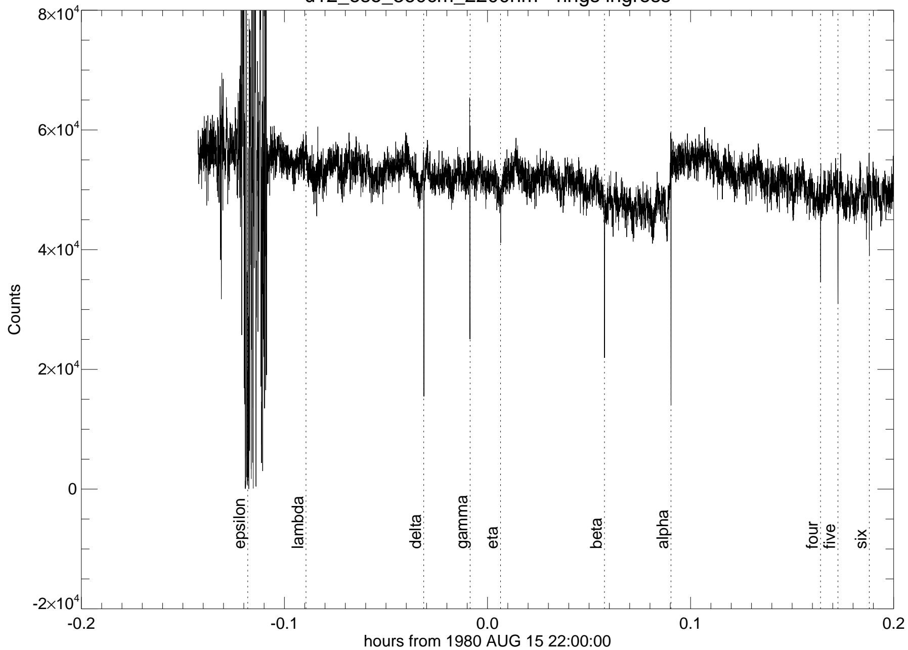
u12_eso_360cm_2200nm - rings ingress
